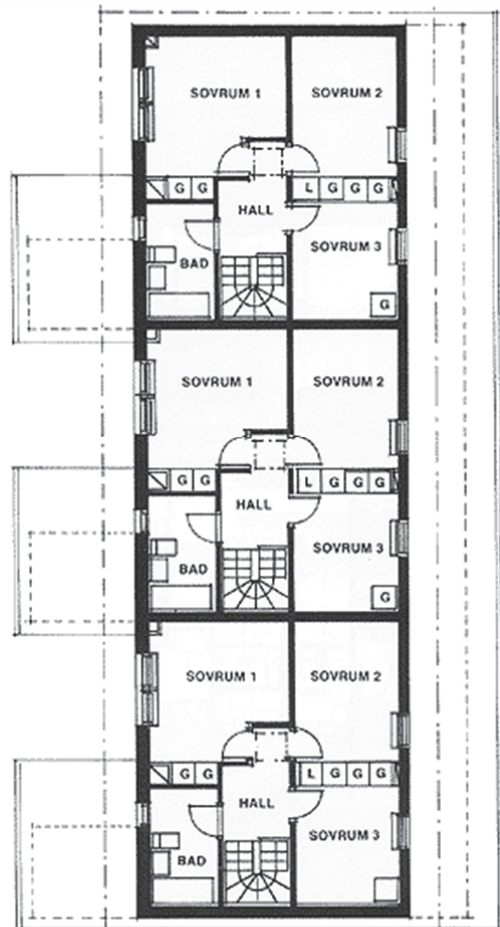
Ovanvåning
